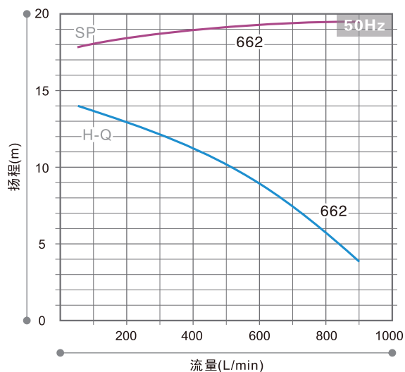
性能曲线图
