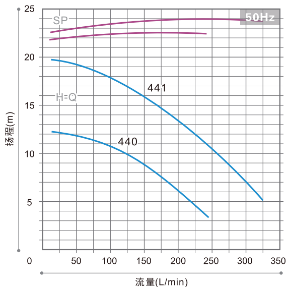
性能曲线图
