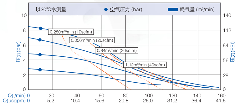
性能曲线图
