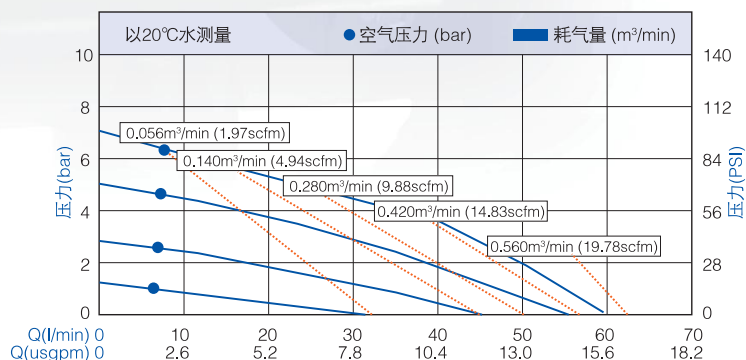
性能曲线图
